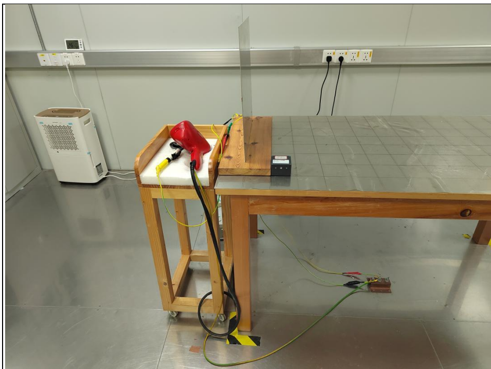
ESD TEST
